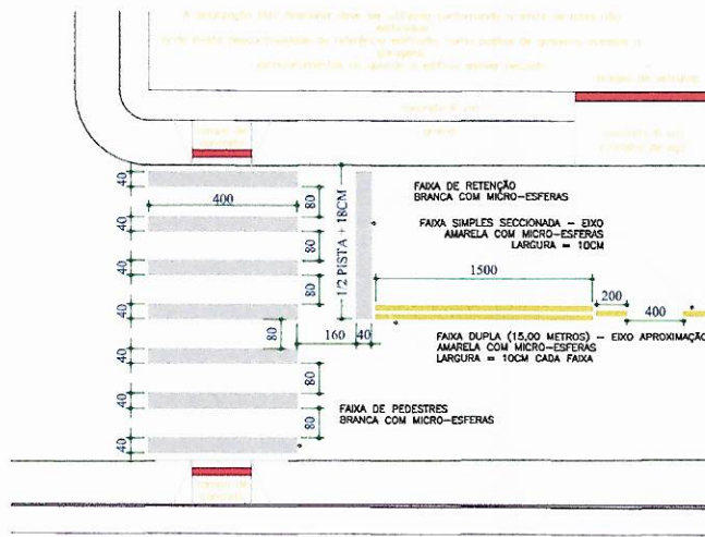
DETALHE GENÉRICO- SINALIZAÇÃO HORIZONTAL SEM ESCALA
